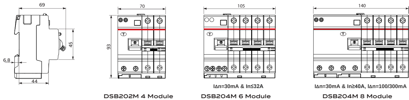
RCBO - DSB200M
